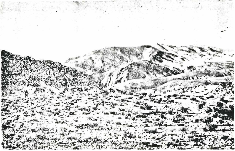
Fot. 7. — El cañón visto desde la superficie de superposición. A la derecha, la sierra Alta y el cerro Galikapor; a la izquierda, el adosamiento de escamas mesozoicas de la sierra del Mal Paso.
