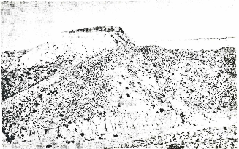
Fot. 12. — La vieja superficie de superposición, recortada por la erosión fluvial cuaternaria.
