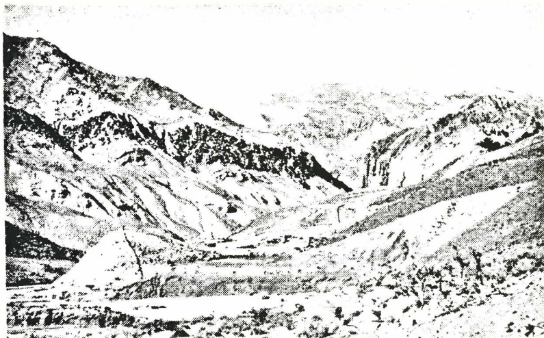
Fot. 3. — El cañón de Yacoraite visto desde el río Laguna.
