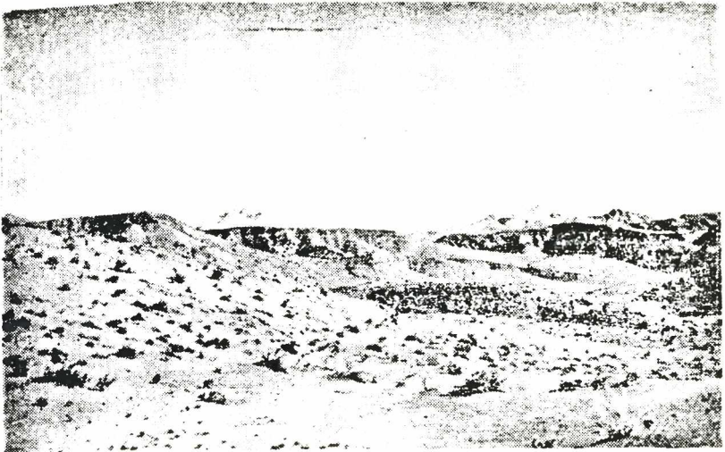
Fig. 10. — Vista hacia el otro flanco del sinclinal precitado; en primer plano, las formaciones de relleno de cuenca, que posibilitaron la sobreimpresión. Al fondo, nevada, la sierra de Aguilar (5.125 m.).
