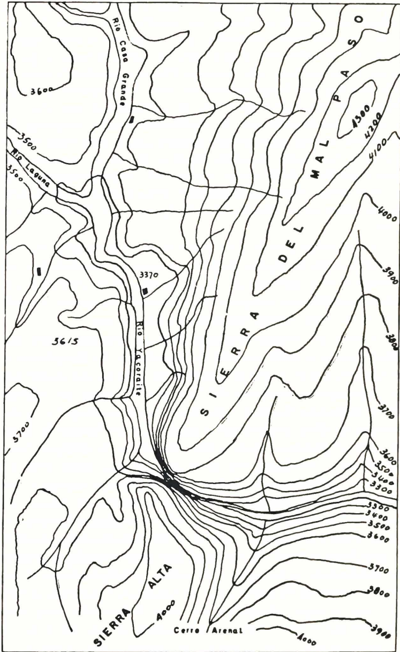
Fig. 4. — Bosquejo topográfico del área del cañón de Yacoraite.
