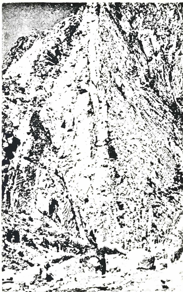
Fot. 5. — El seccionamiento en los estratos verticales de la Formación Yacoraite.
