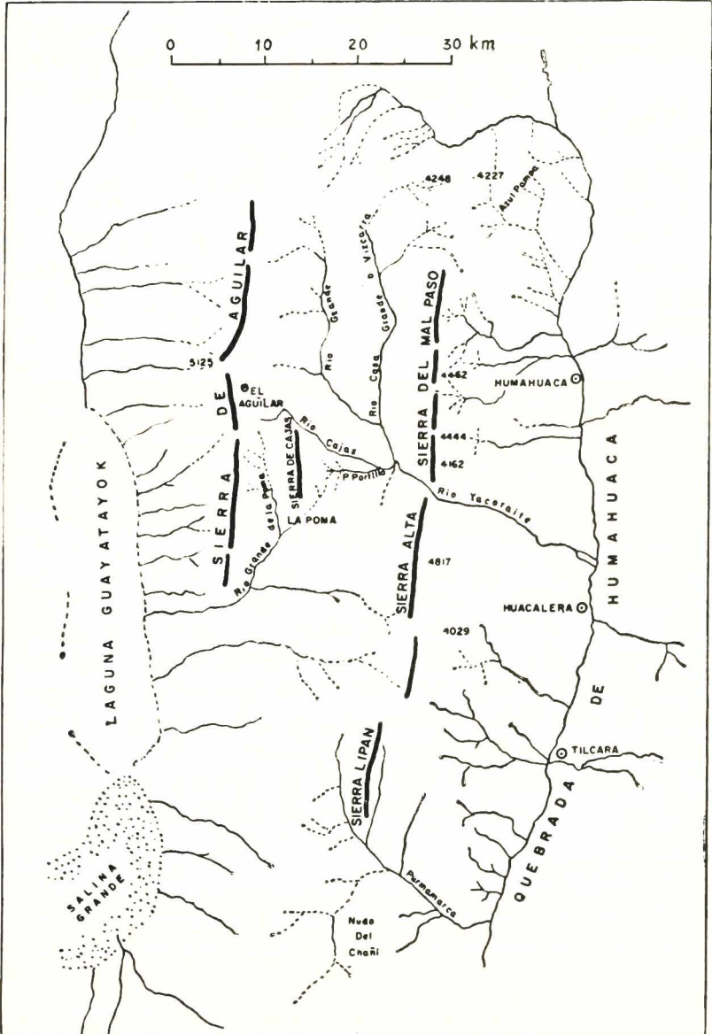
Fig. 1. — Croquis orohidrográfico del borde oriental de la Puna.
