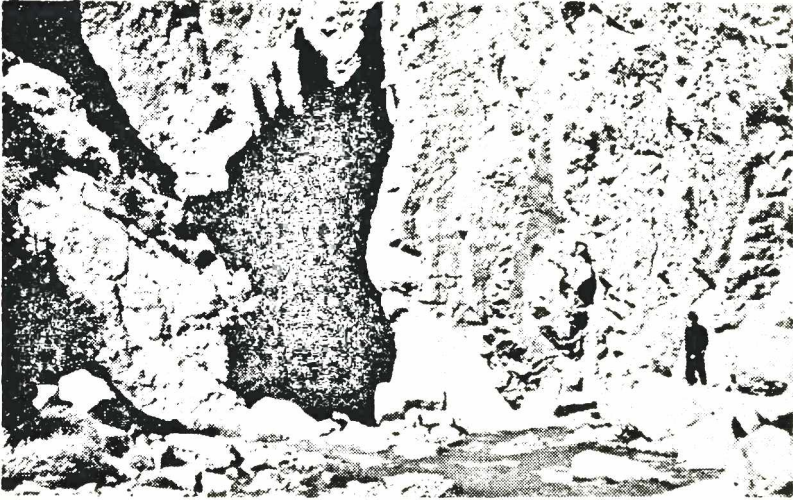
Fot. 6. — Lugar en que el ancho del cañón se reduce a tres metros.
