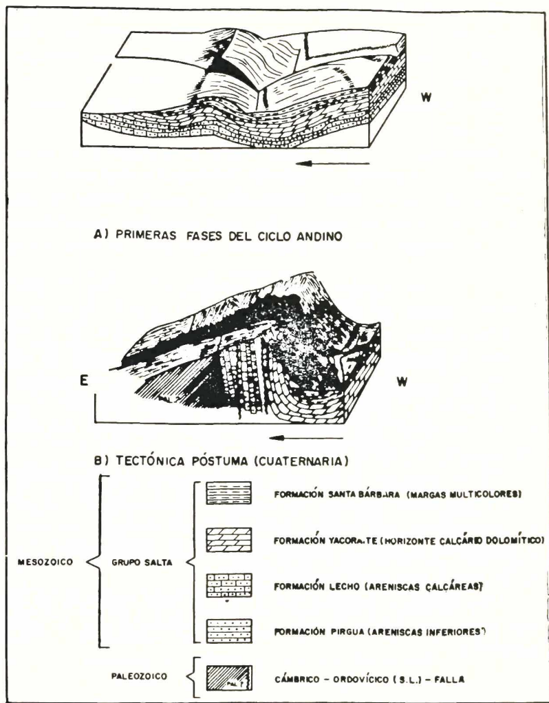
Fig. 2. — Evolución del cañón de Yacoraite.
