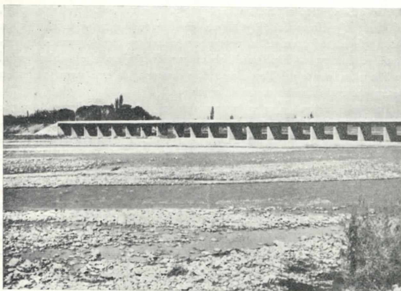
Fot. 4. — Dique Cipolletti, sobre el río Mendoza, en Luján.
