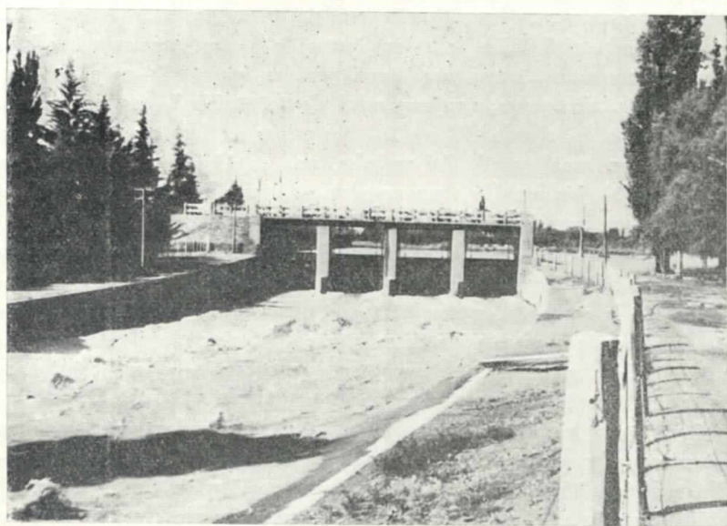
Fot. 5. — El canal Zanjón Cacique Guaymallén a su salida del dique Cipolletti.
